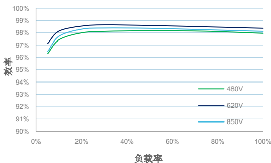
效率曲线
