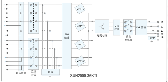
电路框图
